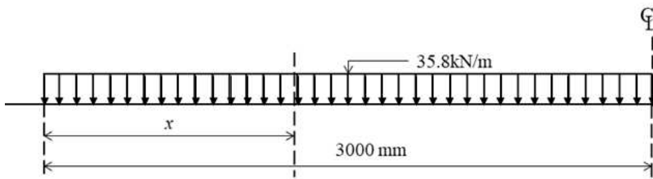
(a) 부재 치수 및 하중 조건
