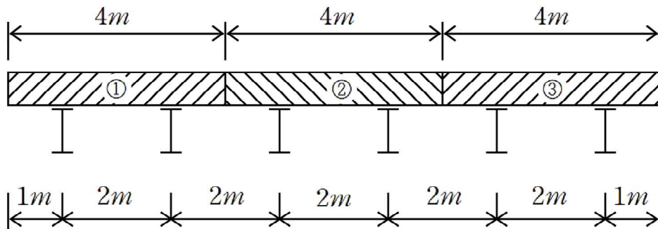
그림 B. 프리캐스트 콘크리트 분절 바닥판 강합성교
